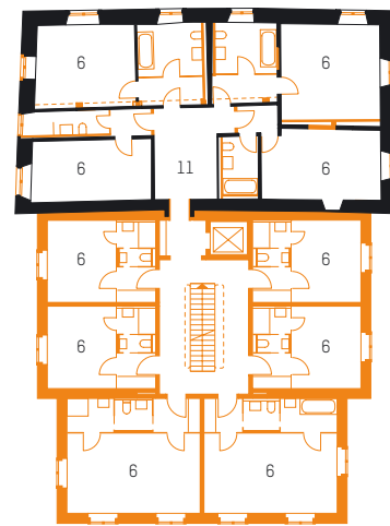
1. Obergeschoss M 1:400
